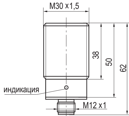
Габаритный чертеж
