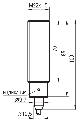
Габаритный чертеж
