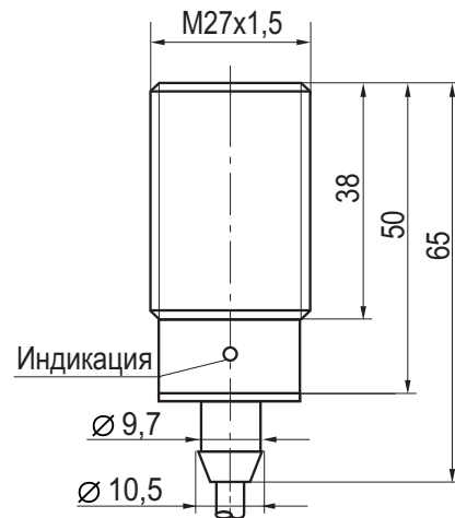
Габаритный чертёж
