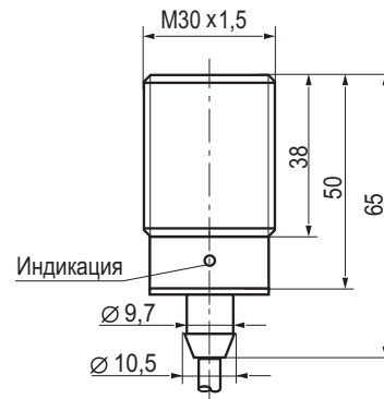
Габаритный чертеж
