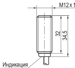
Габаритный чертеж
