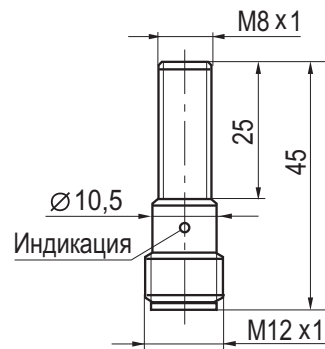
Габаритный чертеж
