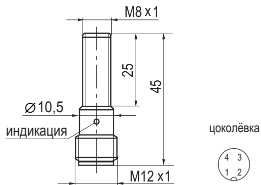
Габаритный чертеж
