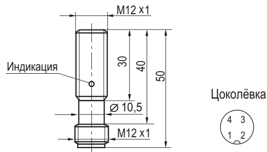
Габаритный чертеж
