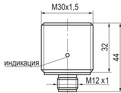
Габаритный чертеж
