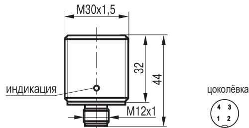
Габаритный чертеж
