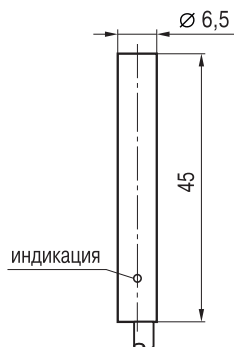
Габаритный чертеж
