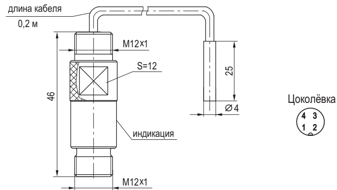
Габаритный чертеж
