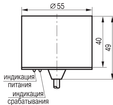
Габаритный чертеж
