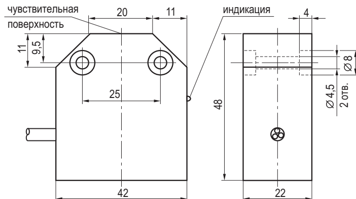
Габаритный чертеж
