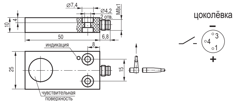
Габаритный чертеж
