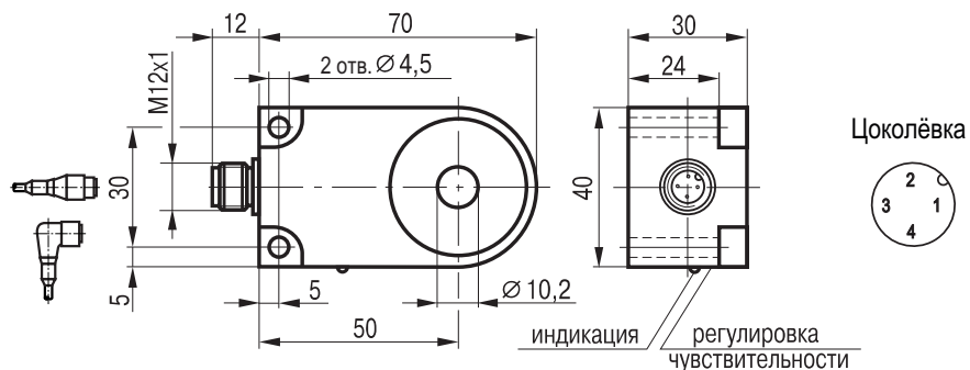
Габаритный чертеж
