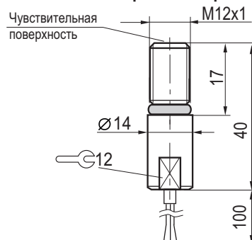
Габаритный чертеж
