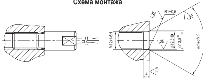
Схема монтажа
