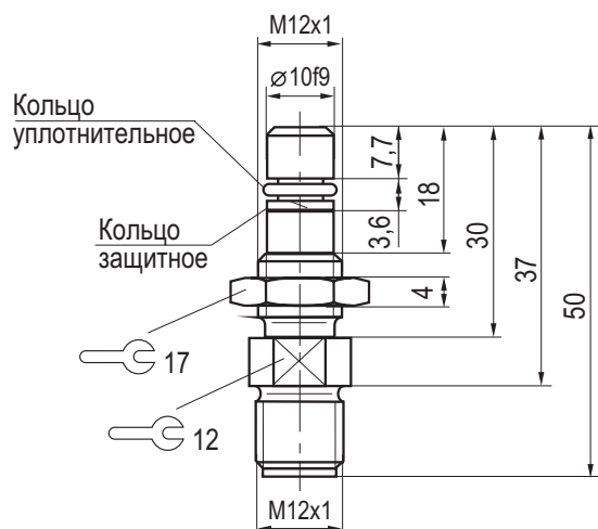
Габаритный чертеж
