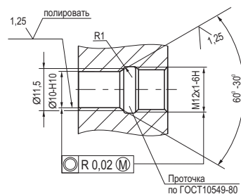
Посадочное место
