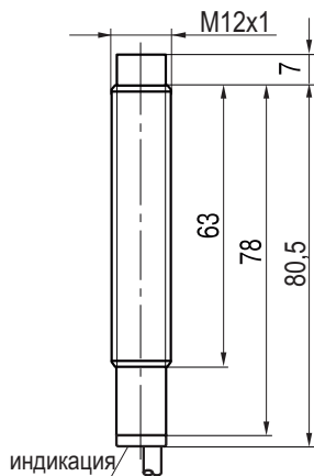
Габаритный чертеж
