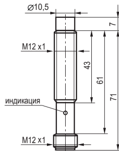
Габаритный чертеж
