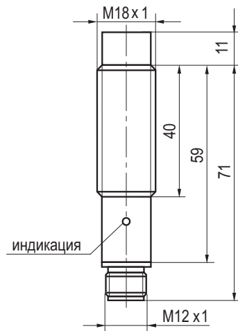
Габаритный чертеж
