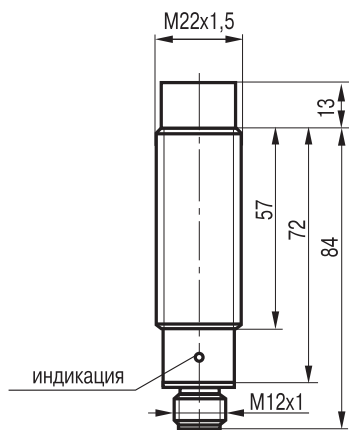
Габаритный чертеж
