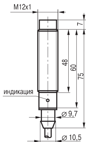
Габаритный чертеж
