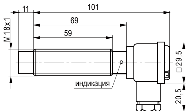
Габаритный чертеж
