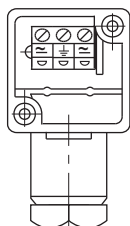
Маркировка клемм
