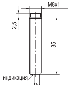
Габаритный чертеж
