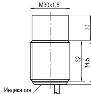
Габаритный чертеж
