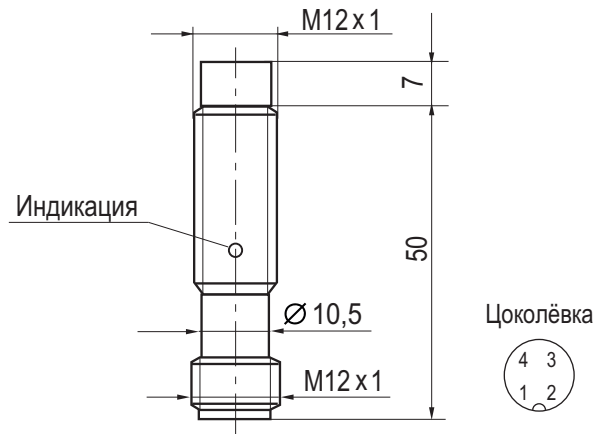
Габаритный чертёж
