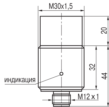
Габаритный чертеж
