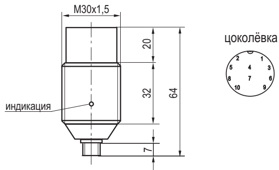
Габаритный чертеж
