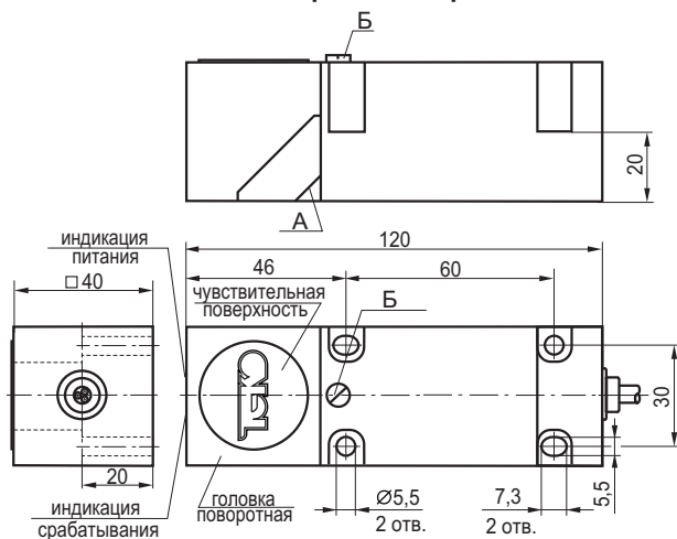
Габаритный чертеж
