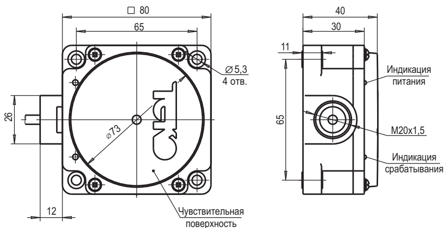
Габаритный чертеж
