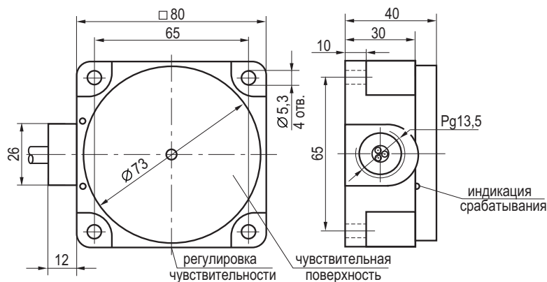
Габаритный чертеж
