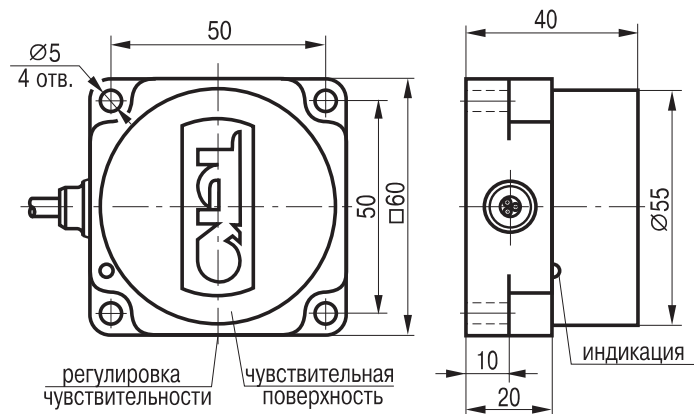
Габаритный чертеж
