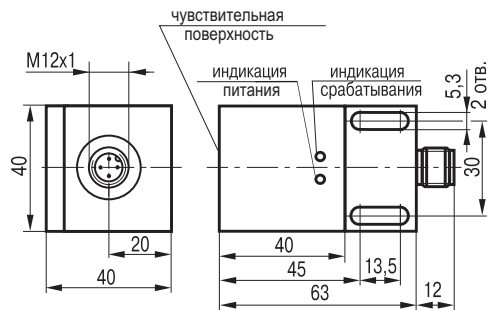
Габаритный чертеж
