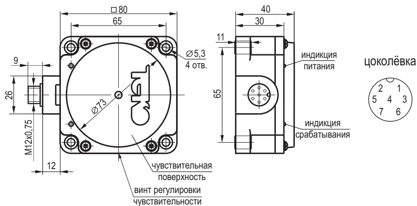
Габаритный чертеж
