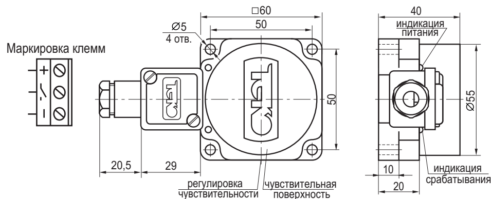
Габаритный чертеж
