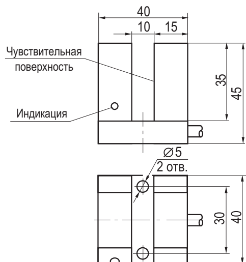
Габаритный чертеж
