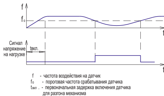
Диаграмма работы
