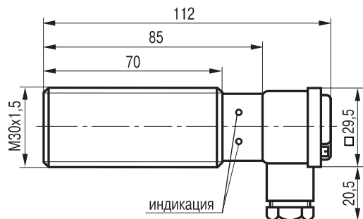
Габаритный чертеж
