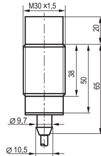
Габаритный чертеж
