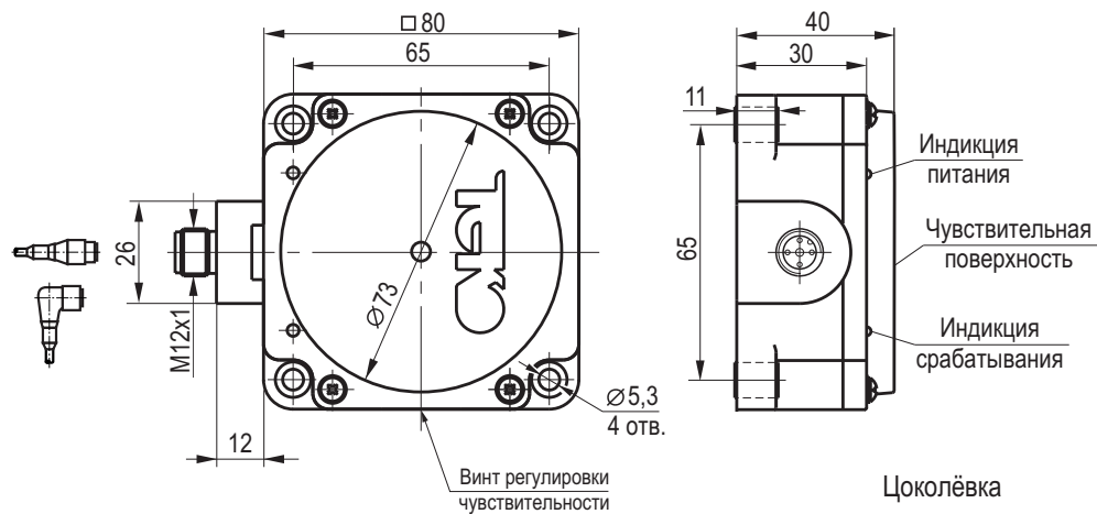
Габаритный чертеж
