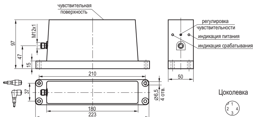
Габаритный чертеж
