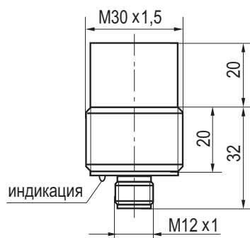
Габаритный чертеж
