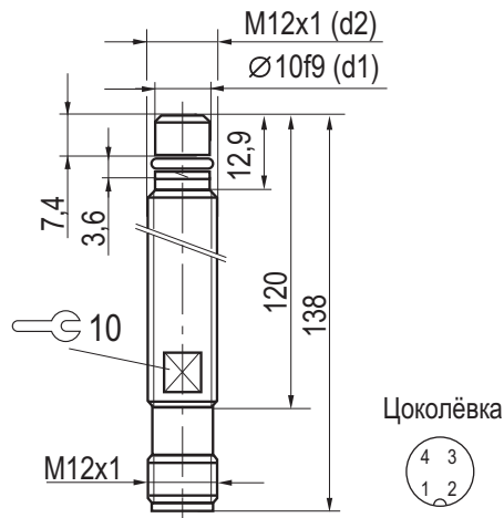
Схема монтажа
