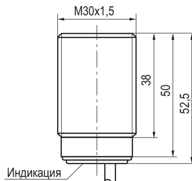
Габаритный чертеж
