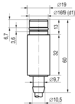
Габаритный чертеж
