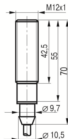
Габаритный чертеж
