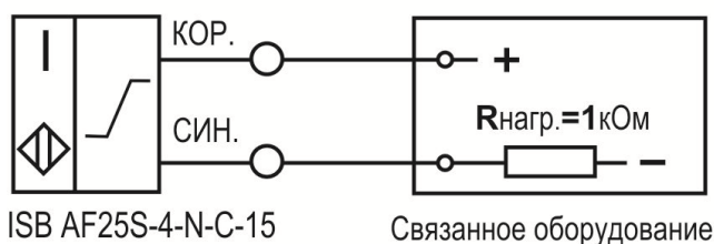
Схема подключения к оборудованию
