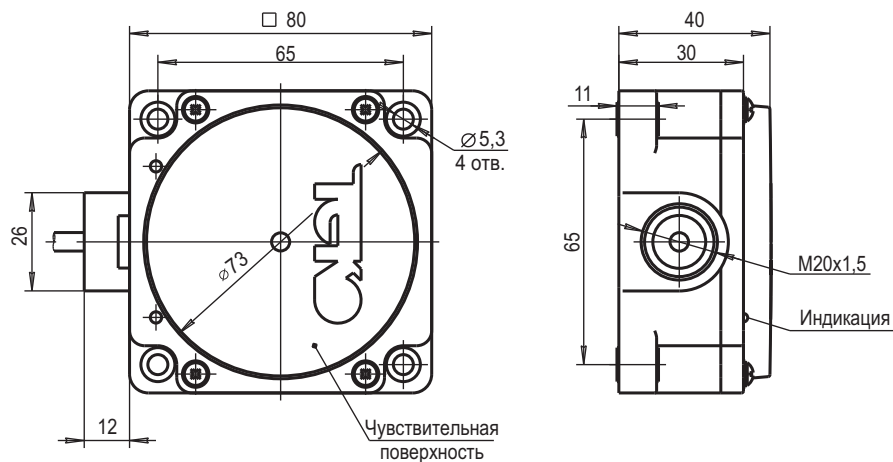
Габаритный чертеж
