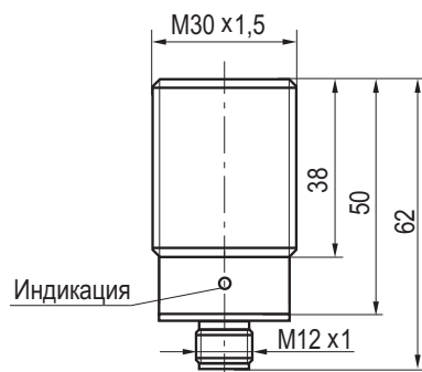
Габаритный чертеж
