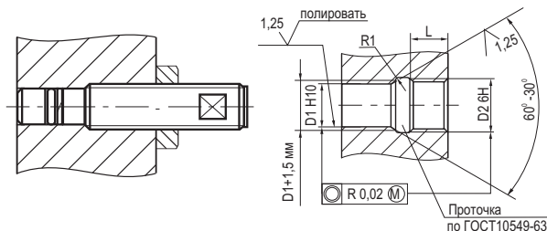
Схема монтажа
